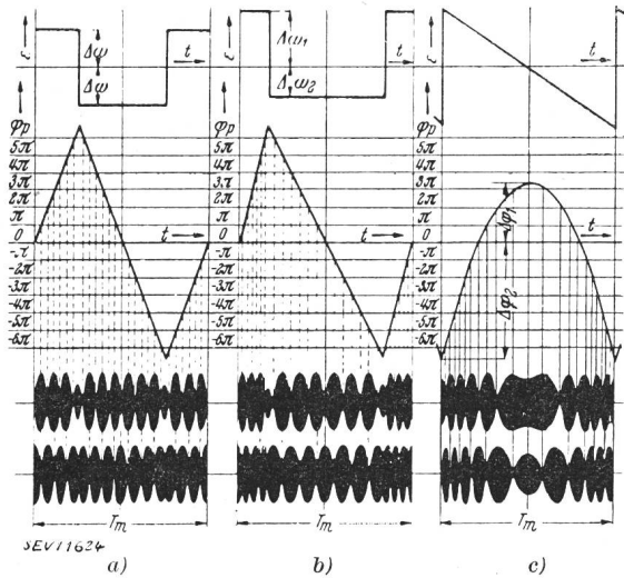
Fig. 4. Schwebungsbilder bei verschiedenen Modulationskurven
