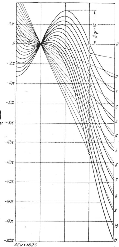
Fig. 5. Phasenwinkelverlauf bei verschiedenen hoher Überlagerungsfrequenz
