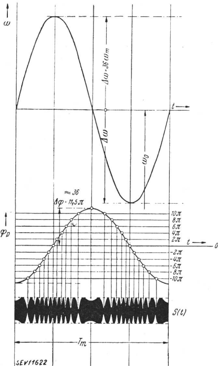
Fig. 2. Entstehung des Schwebungsbildes bei Überlagerung einer frequenzmodulierten Schwingung mit einer Schwingung konstanter Frequenz
