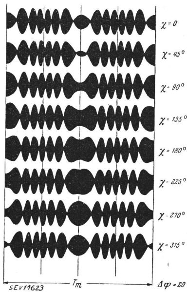
Fig. 3. Schwebungsbilder bei verschiedenen Nullphasenwinkeln
