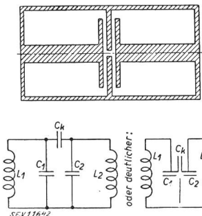
Fig. 3. Kapazitiv gekoppeltes Bandfilter Oben: Schnitt. Unten: Ersatzschema.
