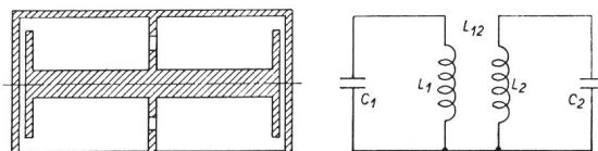
Fig. 4. Induktiv gekoppeltes Bandfilter Links: Schnitt. Rechts: Ersatzschema.
