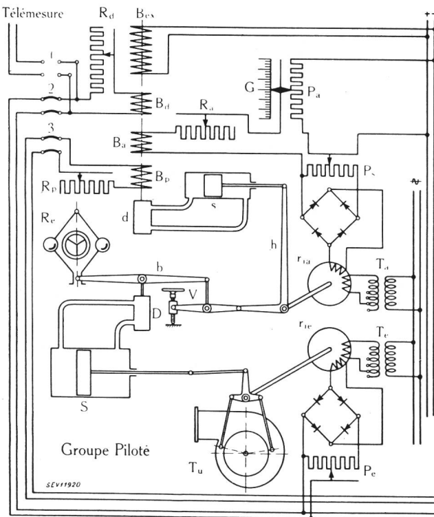
Schéma de deux régulateurs automatiques de vitesses, équipés de dispositifs de réglage fréquence-puissance Brown Boveri-Charmilles
