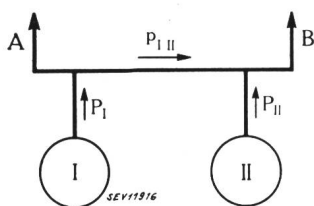
Fig. 2. Fonctionnement en parallèle de deux groupes I et II sur deux réseaux de consommation A et B
