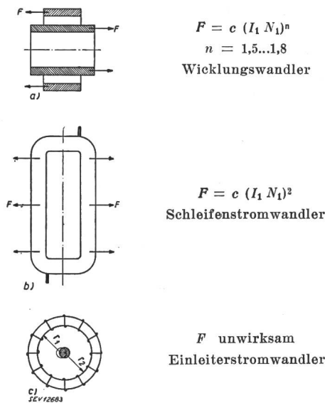
Fig. 3. Kurzschlußkräfte
