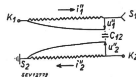
Fig. 9. Répartition de la tension correspondante à l'oscillation du champ de fuite. Couplage étoile/étoile
