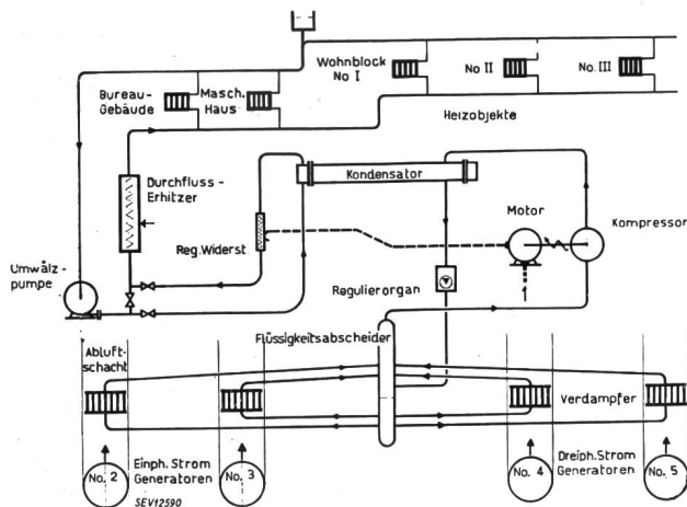
Fig. 2. Schema der Wärmepumpen-Anlage
