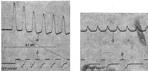
Fig. 3. Wirkungweise des abgestimmten Kontaktes beim Einschalten eines Drehstrom-Transformators von 5 MVA a Einschaltstrom des Transformators b Einschaltimpulse auf die Spule des Zeitschützes
