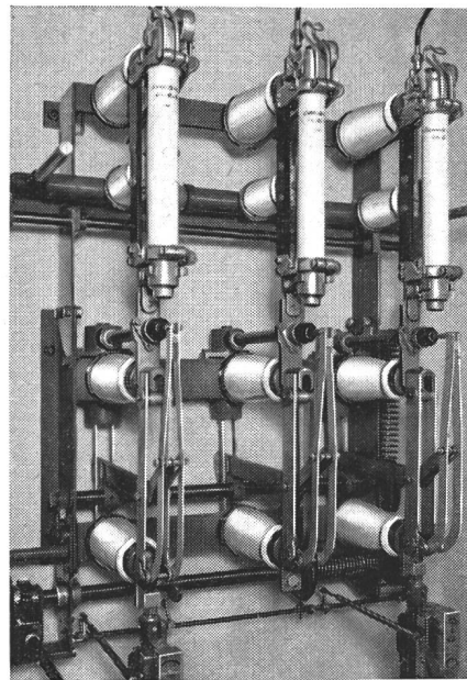
Fig. 2. Sectionneur auto-pneumatique de charge 20 kV, 150 et 400 A, combiné avec un coupe-circuit tripolaire
