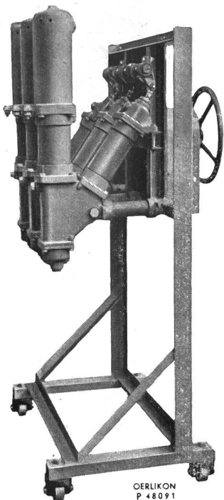
Fig. 3. Oelarmierter Schnellschalter, Typ V-4 600 A, 10 kV, Abschaltleistung 250 MVA
