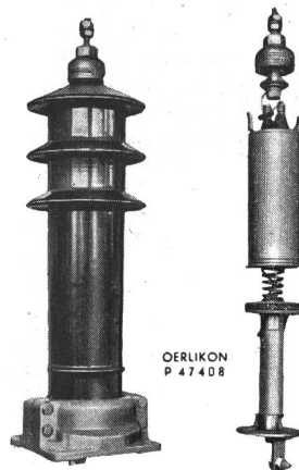
Fig. 4. Kondensator-Ueberspannungsableiter
