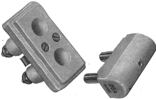
Fig. 5. Coupe-circuit à broches Gardy pour tableaux
