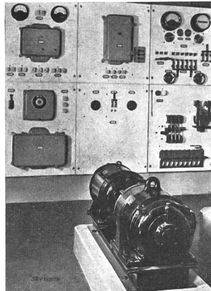
Fig. 1. Drehstrom-Notstromgruppe 15 kVA, 3x220 V, durch Gleichstrommotor angetrieben, mit automatischer Anlassvorrichtung
