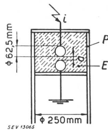
Fig. 35. Gefäß für Durchschlagmessungen
