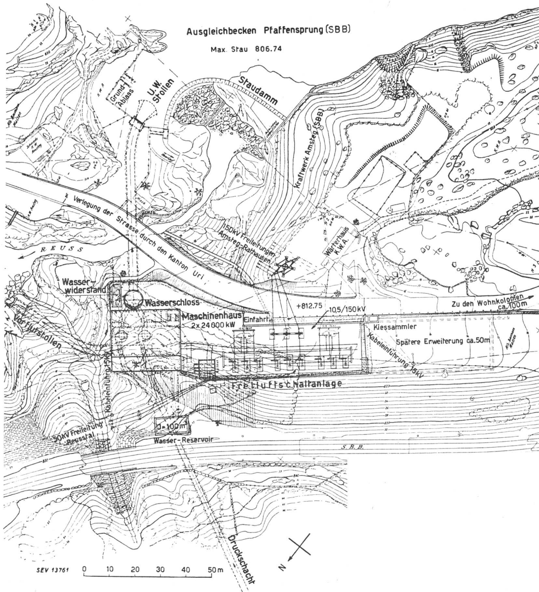
Fig. 5. Maschinenhaus Wassen, Situationsplan
