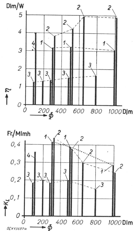
Fig. 5. Mittlere Lichtausbeute \eta in Dlm/W und Lampenkosten K_L pro Mlmh verschiedener Lampentypen, abhängig vom Nennlichtstrom \Phi . 1 Hg-Entladungs-Lampe; 2 Na-Entladungs-Lampe; 3 Glühlampen Dlm-Reihe, 220 V; 4 Niederspannungs-Fluoreszenzlampe (Typ «weiss»)
