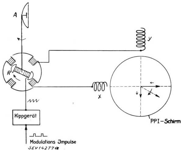
Fig. 7 Die PPI-Aufzeichnungsmethode (Erläuterungen im Text)
