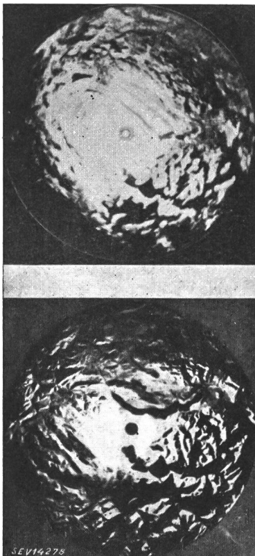
Fig. 8 Vergleich eines PPI-Schirmbildes (oben) mit dem entsprechenden Relief bei analoger Ausleuchtung (unten)
