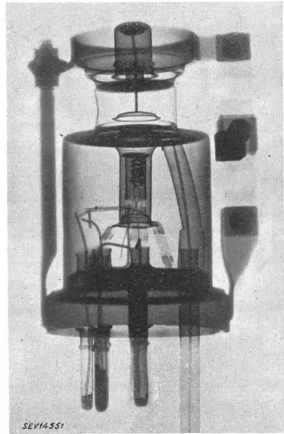
Fig. 9 Röntgenaufnahme eines Klystrons (Reflexionsklystron Typ 723 A/B) Betriebswellenlänge \lambda = 3 \text{ cm} , Wirkungsgrad \mu = 4 \%
