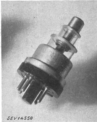
Fig. 7 Sendetriode Typ RCA 2C43 Betriebswellenlänge \lambda = 10 \text{ cm} Dauerleistung 1 W
