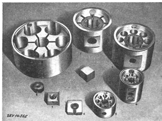
Fig. 3b Anodensysteme moderner amerikanischer Magnetrons ? Anodensystem eines Schlitzmagnetrons, bei den anderen ab- gebildeten Systemen erkennt man die Bildung ausgeprägter Induktivitäten und Kapazitäten
