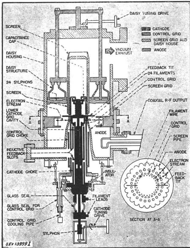
Fig. 8 Schnitt durch ein Resatron Betriebswellenlänge \lambda = 50 \text{ cm} , Dauerleistung 50 kW
