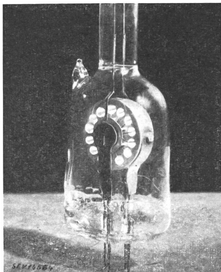
Fig. 3a Versuchsmagnetron mit Sternverbindung der gleichphasigen Anodensegmente (aus der vor einigen Jahren in der Schweiz begonnenen Entwicklung)
