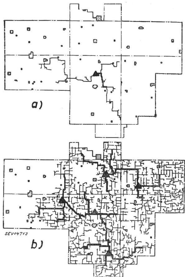
Fig. 2 Beispiel eines landwirtschaftlichen Netzes einer Genossenschaft a) Zustand 1936 mit 203 Abonnenten b) Endausbau mit 5600 Abonnenten — dreiphasige Leitung — einphasige Leitung ▲ Transformatorstation
