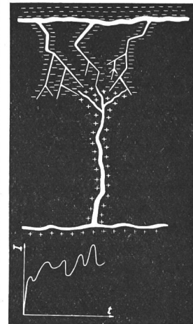
Fig. 18 Uebergang zum quasi-stationären Zustand des Blitzstromes
