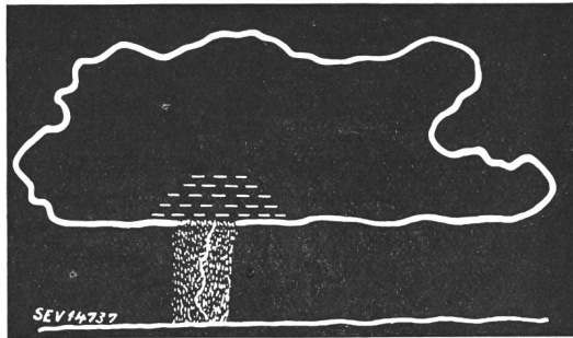
Fig. 16 Einleitende Entwicklung eines Blitzes von einer negativ geladenen Wolke zur Erde
