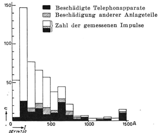
Fig. 9 Störströme in A auf schwedischen Telephonleitungen im Jahre 1943
