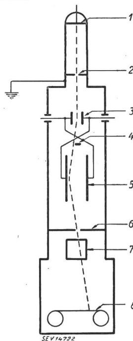
Fig. 1 Vom Verfasser entwickelte Schaltung des Kathodenstrahl-Oszillographen für 40 kV Gleichspannung 1 Kathode 2 Anodenöffnung 3 Ablenkplatten 4 Sperrelektrode 5 Ablenkplatten 6 Schirmplatte 7 Zeitkreisplatte 8 Film
