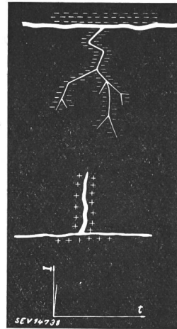
Fig. 17 Beginn der Hauptentladung eines Blitzes aus einer negativ geladenen Wolke zur Erde
