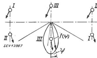
Nebenbündelfreie Richtstrahleranordnung mit der Kennlinie f(\psi) = (1-\psi^2)^{5/2}
