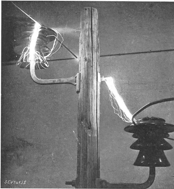
Fig. 5 Trockenüberschlag am Mastkopf 270 kV 70 cm Stützenabstand (Gemmileitung)
