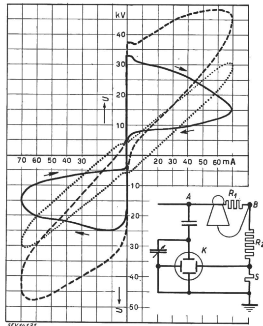
Fig. 1 Lichtbogen Pol-Erde über Isolator und nasse Stange Die Spannung am Isolator steigt bis 33 kV, der Lichtbogen zündet und die Lichtbogenspannung fällt bis zum Nulldurchgang. In der andern Phase der Wechselfspannung ist der Verlauf symmetrisch.
