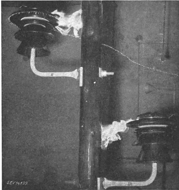
Fig. 9 Ueberschlag unter Regen 155 kV
