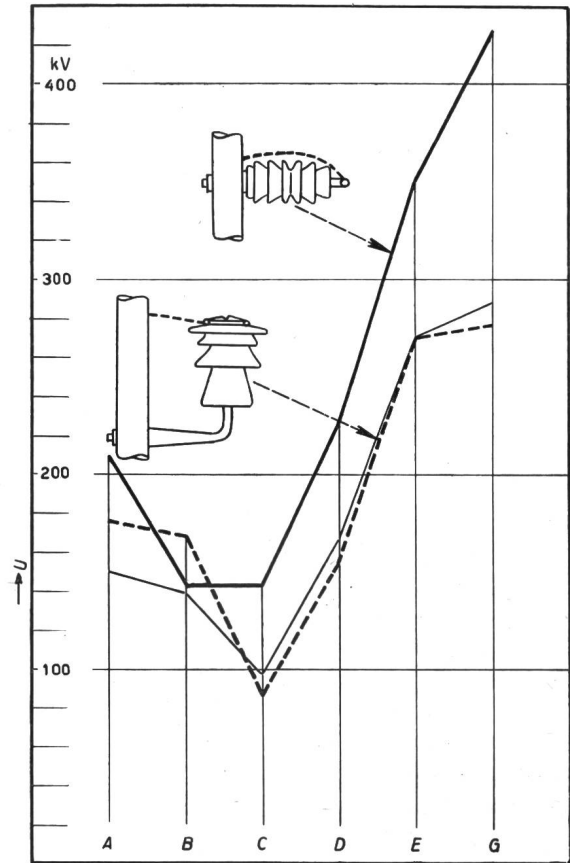
Fig. 11 Ueberschlagswerte in verschiedener Anordnung A trocken auf gerader Stütze; B nass auf gerader Stütze; C nass, ein Isolator am Mast; D nass von Leiter zu Leiter am Mast; E trocken von Leiter zu Leiter am Mast; G 50 % minimale Ueberschlag-Stoßspannung von Leiter zu Leiter, reduziert um \frac{1}{\sqrt{2}}
