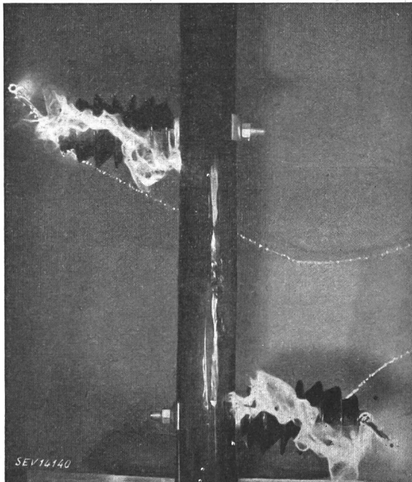
Fig. 10 Ueberschlag unter Regen 226 kV
