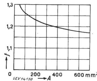
Fig. 9 Einfluss des Windes auf die Belastbarkeit der Freileitungen f Korrekturfaktor für eine Windgeschwindigkeit v = 0,6 m/s (nach Frick); A Leiterquerschnitt.
