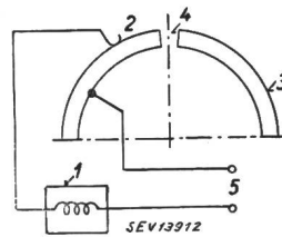
Fig. 39 Schematischer Aufbau einer Abstimmung mit Motor 1 Motor. 2 Kontakt 3 Kontaktbahn 4 Schlitz. 5 Netzanschlussklemmen
