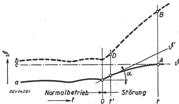
Fig. 1 Wirkungsweise von Temperatur-Signalgeräten a Temperaturverlauf am Einbauort des Signalgerätes b Temperaturverlauf am Verlustherd c Einstellwert eines Thermokontaktes θ' Einstellwert eines Temperaturgradient-Signalgerätes
