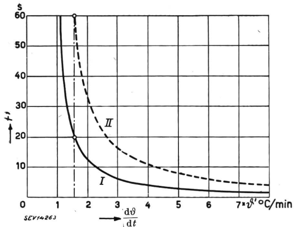
Fig. 3 Anspruchzeit t' in Funktion der Temperaturanstiegsgeschwindigkeit \frac{d\theta}{dt}
