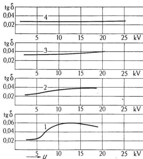
Fig. 6 Spannungsabhängigkeit des Verlustfaktors verschiedener Nut-Isolationen
