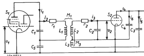
Fig. 2 Schaltbild eines rückgekoppelten Bandfilters
