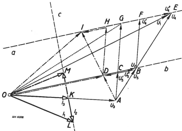
Fig. 3 Vektordiagramm der Teilspannungen eines magnetischen Stabilisators punktierte Vektoren: Resonanzfall strichpunktierte Vektoren: Netzspannung zu tief vollausgezogene Vektoren: Netzspannung zu hoch a geometrischer Ort der Spitze von U_1 ; b konstante Richtung von U_2 ; c geometrischer Ort von I_2
