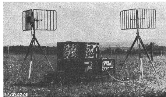
Fig. 8 Tragbares Dezimeterwellen-Gerät mit Mehrkanal-Zusatz von links nach rechts: Antenne mit angebautem Sender; Armeetelephon; Mehrkanal-Zusatz für 2 Telephonie- und 2 Telegraphiekanäle mit Leitungsnachbildungen; Dezimeterwellen-Gerät; Gleichrichter; Empfangsantenne
