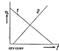
Fig. 15 Einstelldiagramm für zweiseitige, frequenzabhängige Regelung der Übergabeleistung
