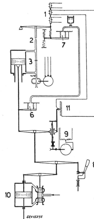
Fig. 10 Schema des Reglers für konstante Maschinenleistung innerhalb eines schmalen Frequenzbandes Leistungsregler 1 Leistungsmeßsystem 2 Ventil 3 Servomotor 6 Geber- und 7 Empfängerbalg für Temporärstatik Drehzahlregler 8 Pendel 9 Leistungseinstell- vorrichtung 10 Hauptservomotor 11 Potentiometer zur Nachsteuerung des Leistungsreglers
