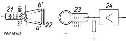
Fig. 5 Nachfokussiergerät
