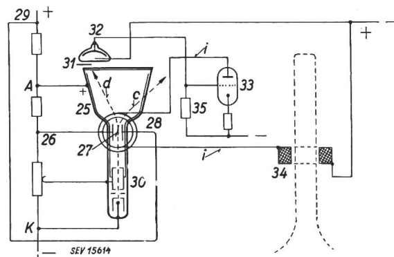
Fig. 6 Regler für die Fleckschärfe
