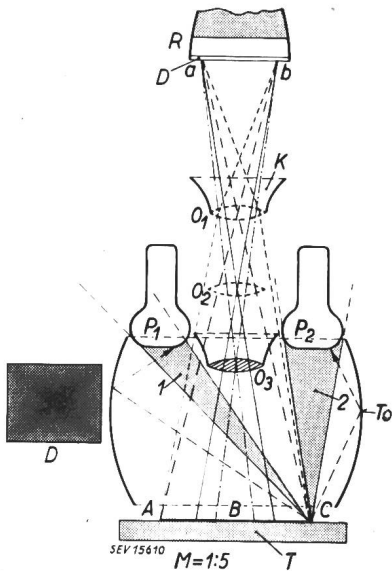
Fig. 2 Abtastoptik f -Werte: \theta_1 133,3 mm; \theta_2 150,0 mm; \theta_3 133,3 mm; Die optische Durchlässigkeit des Transparentes D ist nach beiden Koordinatenrichtungen so abgetönt, dass für jeden Bildpunkt das Produkt aus \sigma und dem zugehörigen Wert aus Fig. 2a konstant ist. (Das im Bild D erscheinende Schattenkreuz beruht auf einem Fehler im Klischee; die Helligkeit nimmt von der Bildmitte aus nach den Rändern gleichmässig zu.)
