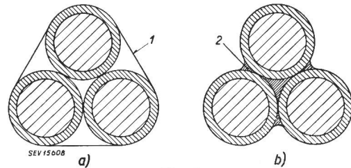
Fig. 2 Bündelung der Schweisselectroden 1 Papierband; 2 Umhüllungsmasse
