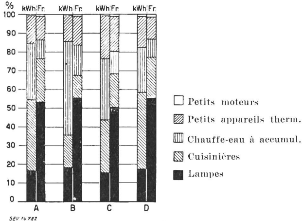
SEV 14782 Fig. 9 Répartition de la consommation et des recettes des appareils électro-domestiques, en 1945, selon les catégories d'entreprises électriques
