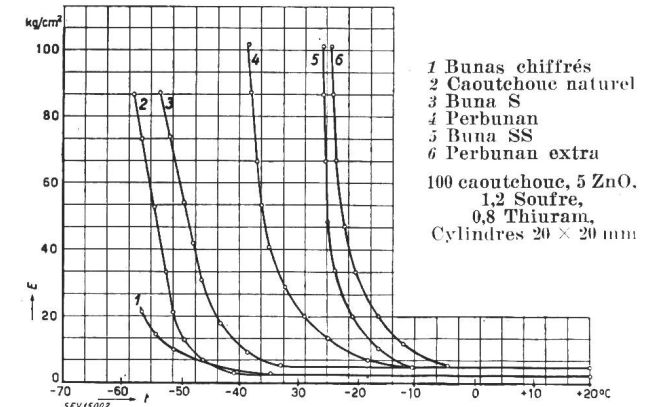
Fig. 2 Module d'élasticité (E) des caoutchoucs naturel et synthétiques en fonction de la température (t) 1 Bunas chiffrés, 2 Caoutchouc naturel, 3 Buna S, 4 Perbunan, 5 Buna SS, 6 Perbunan extra 100 caoutchouc, 5 ZnO, 1,2 Soufre, 0,8 Thiuram, Cylindres 20 x 20 mm
