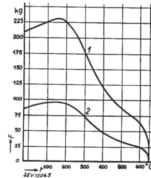
Fig. 5 Résistance à la traction d'un ruban Largeur: 25 mm Épaisseur: 0,25 mm 1 Fibres continues, 2 Fibres discontinues, F force, t température
