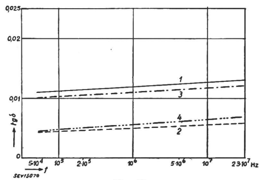
Fig. 10 Pertes diélectriques
