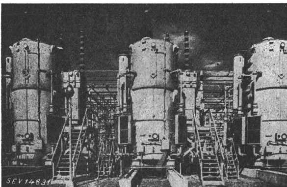
Fig. 6 Transformatorengruppe von 3 x 50 000 kVA 220/66 kV mit Stufenschaltern
