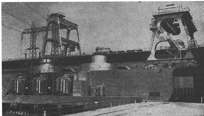
Fig. 5 Ansicht der Freiluftgeneratoren des Wheeler-Kraftwerkes der TVA [2 (4) x 36 000 kVA]
