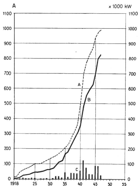
Fig. 2 Entwicklung der Elektrokesselanlagen A Zahl der Betriebe mit Elektrokesseln, je am Jahresende B Installierte Leistung, je am Jahresende C Jährliche Zunahme der installierten Leistung
