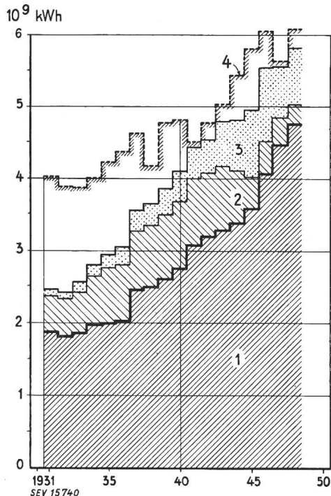
Fig. 1 Der Anteil der Elektrokessel bei der Verwendung der Sommerenergie 1 Inlandverbrauch ohne Elektrokessel 2 Energieausfuhr 3 Energieverbrauch der Elektrokessel 4 Technisch mögliche Energieproduktion
