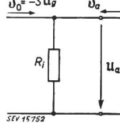
Fig. 5 Ersatzschaltbild für den Anodenkreis einer Röhre eingepprägter Strom
