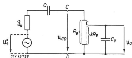
Fig. 12 Endgültiges Ersatzschaltbild
