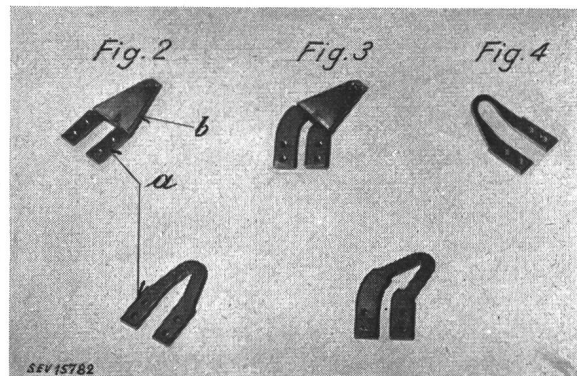
Fig. 2 Lötspitze Typ LP 1 a Heizelement b Lötspitzenmaterial
