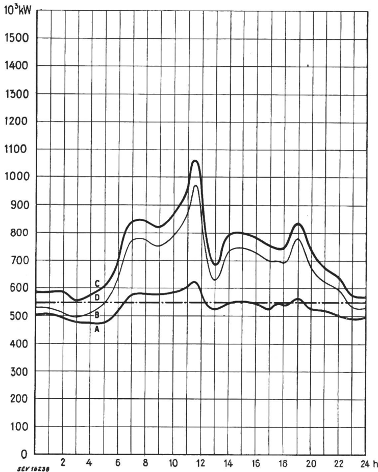
Diagramme de charge journalier du mercredi 16 mars 1949
