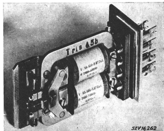
Fig. 10 Polarisiertes Relais mit Isolationen aus Hartpapier
