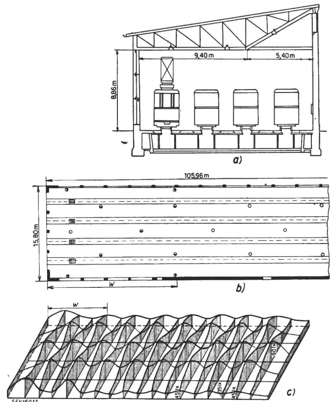
Fig. 1 Beleuchtung einer Wagenhalle a) Aufriss im Schnitt b) Grundriss c) Lichtverteilung über dem Grundriss W Waschplatz o Glockenspiegel • Zonenspiegel ● Schrägstrahler
