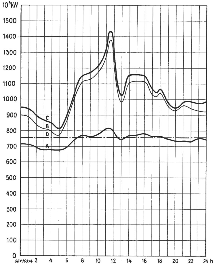
Diagramme de charge journalier du mercredi 18 mai 1949
