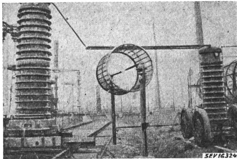
Fig. 1 Kleine «Messreue» Links Prüftransformator Rechts Spannungswandler Versuchsleiter teilweise abgeschirmt
