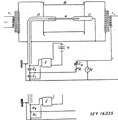
Fig. 2 Schema der kleinen Messreue A Versuchsleiter; B Drahtgeflechtzylinder; D Abschirmung; E Verstärker; T Prüftransformator; T 2 Messwandler; Y Oszillograph
