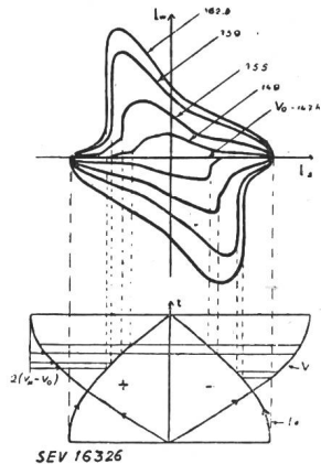
Fig. 3 Stromoszillogramme bei verschiedenen Spannungen Abszisse: Blindstrom Ordinate: Wirkstrom in stark vergrössertem Maßstab Unten die zwei Viertelswellen des Blindstromes (wenn sein Absolutwert abnimmt), und der Spannung (wenn ihr Absolutwert zunimmt), zur Festlegung der Punkte einsetzender Ionisierung ( u_1 ). Es zeigt sich, dass die Gleichung gilt: u_0 - u_1 = u_{\text{max}} - u_0
