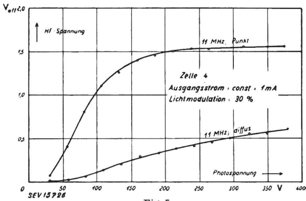
Fig. 5. Ausgangswechselspannung am Vervielfacher in Funktion der Photospannung
