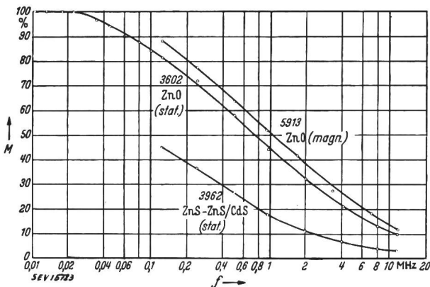
Fig. 2 Frequenzgang der Modulationsfähigkeit U_a = 25 \text{ kV} M Modulationsfähigkeit
