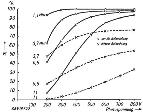
Fig. 6. Verlauf der Strommodulation in Funktion der Beschleunigungsspannung. Modulationsgrad des Photostromes für M Licht = 100 % Kugeldurchmesser 20 cm Ausgangsstrom 1 mA (konstant)
