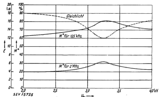
Fig. 4 Abhängigkeit der Modulationsfähigkeit und des Gleichlichtes von der Elektronenlinsenspannung U_{a1} Elektronenlinsenspannung U_{a2} Anodenspannung ( 25 \text{ kV} , mit Raster) I_z Beleuchtungsstärke M^* Modulationsfähigkeit
