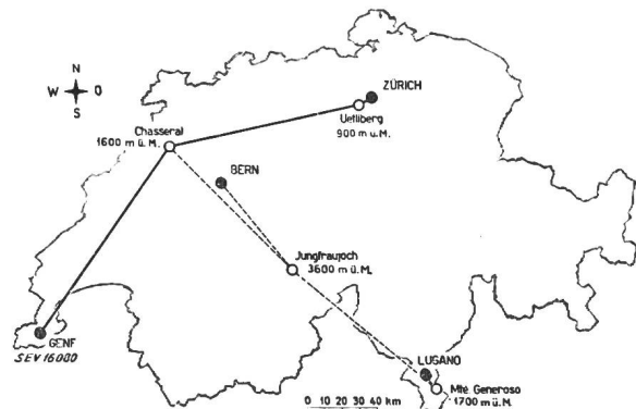
Fig. 1 Richtstrahl-Mehrkanalverbindung in der Schweiz — Verbindung im Betrieb --- Versuchsverbindung ● Endamt ○ Relaisstation
