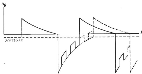
Fig. 3 Kippschwingungen eines gesteuerten Multivibrators
