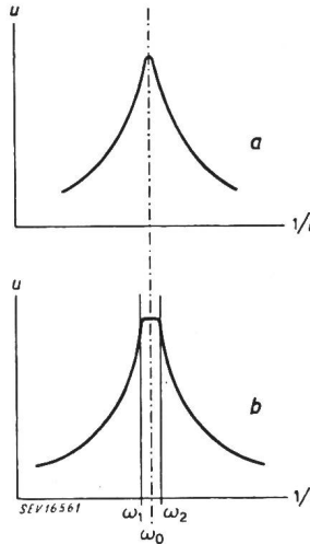
Fig. 5 Resonanzkurve eines Schwingkreises a ohne Dämpfung b bei indirekter Dämpfung \omega_0 Grundfrequenz
