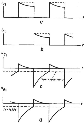
Fig. 2 Kippschwingungen eines freischwingenden Multivibrators a, b Verlauf der Anodenströme c, d Verlauf der Gitterspannungen
