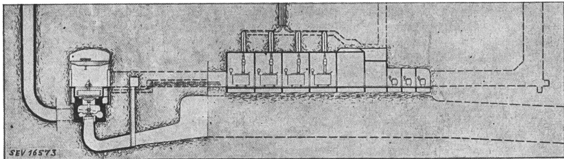
Fig. 3 Querschnitt durch das unterirdische Maschinenhaus des Kraftwerkes Harspränget
