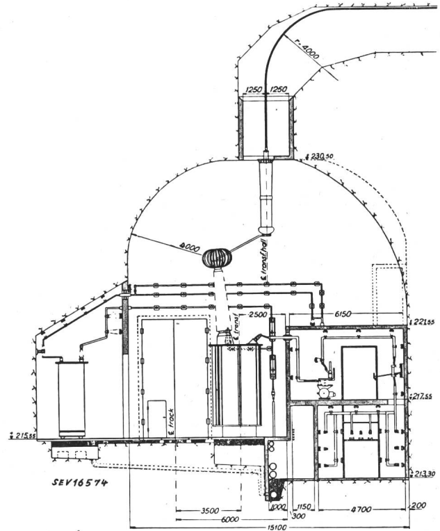
Fig. 4 Querschnitt durch die Transformatorenhalle des Kraftwerkes Harspränget
