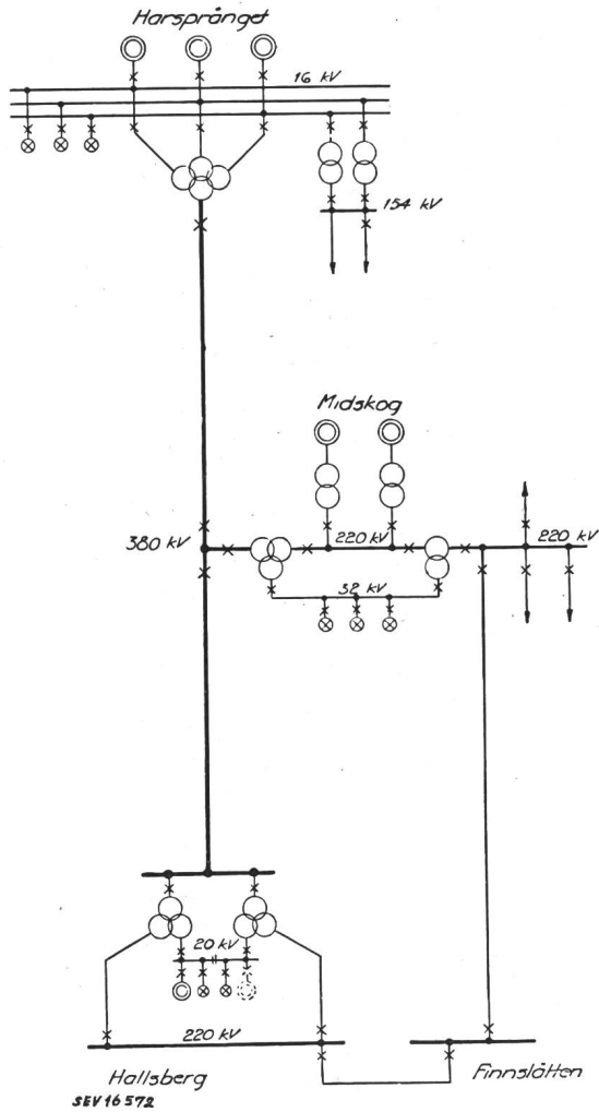
Fig. 2 Schema der geplanten 380-kV-Fernleitung
