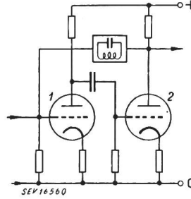
Fig. 4 Zweistufiger Verstärker mit Resonanzrückkopplung
