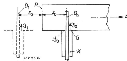
Fig. 8 Hohlleiter mit einem metallisch abgeschlossenen Ende Z_0 Antennenwiderstand im Fusspunkt Z_1 Strom im Spiegelbild R Reflektierende Wand
