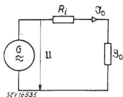
Fig. 7 Elektrisches Ersatzschema für einen Dipol Z_0 Antennenwiderstand im Fusspunkt U Generatorspannung Z_0 Antennenwiderstand des Dipols R_i Innenwiderstand des Generators
