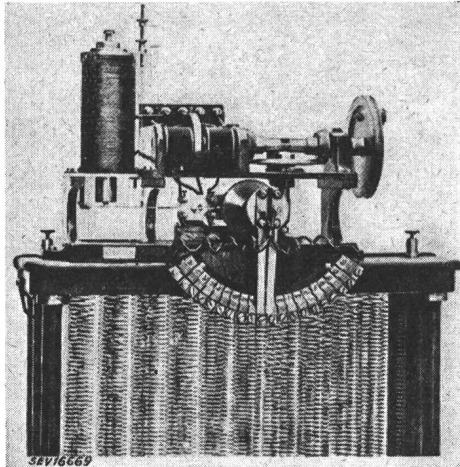
Fig. 9 Régulateur Thury 1 re manière
