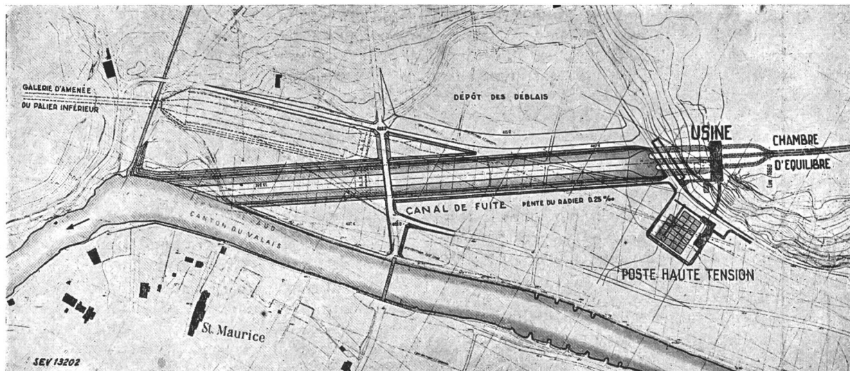
Fig. 27 Lavey Plan de situation de la région de l'usine
