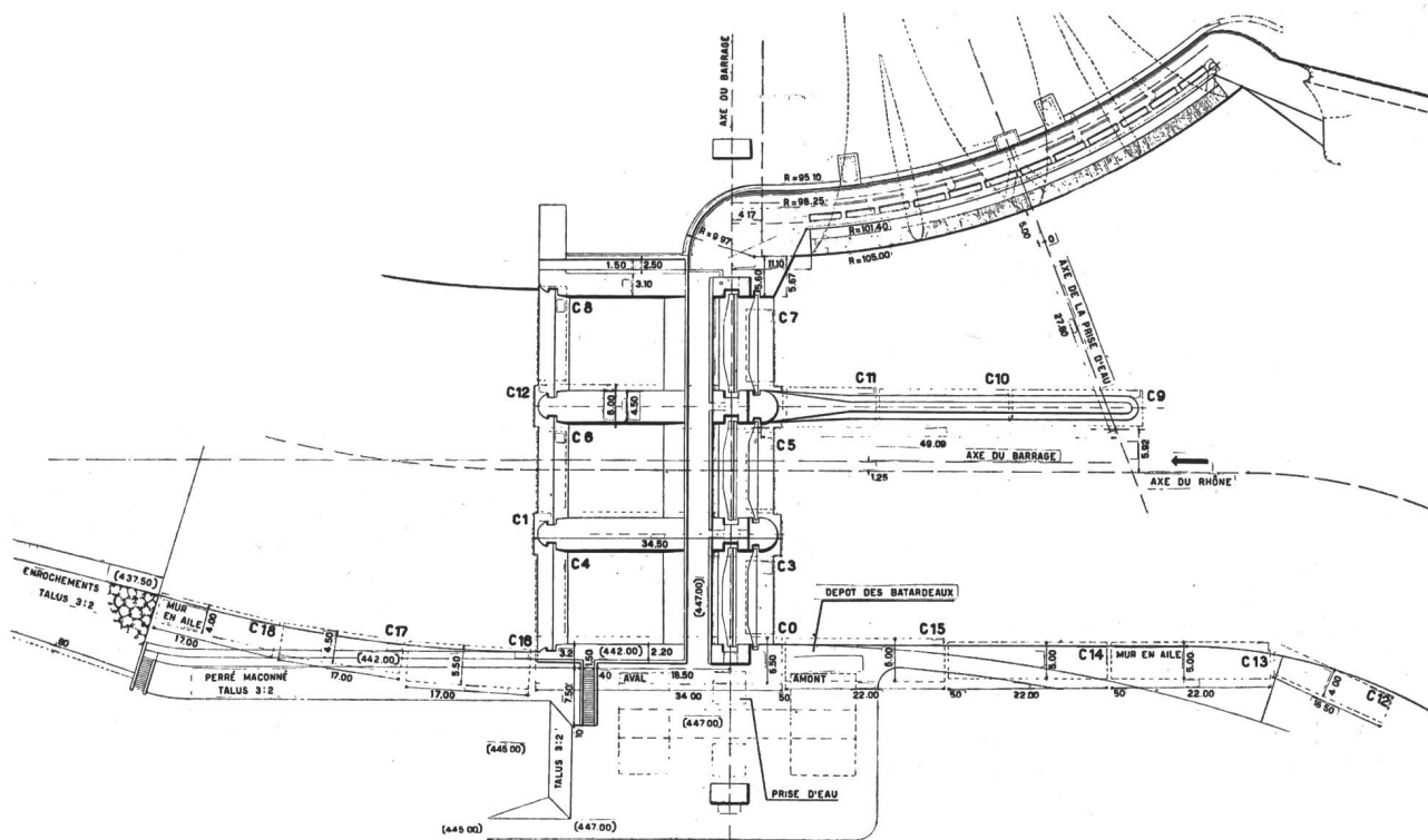
Fig. 21 Lavey Plan de situation du barrage et de la prise d'eau
