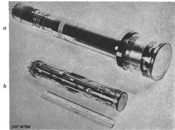
Fig. 8 Fernseh-Kameraröhren a RCA-2P23 Image-Orthicon-Röhre b «Mimo»-Kleinkameraröhre (RCA-2P22)
