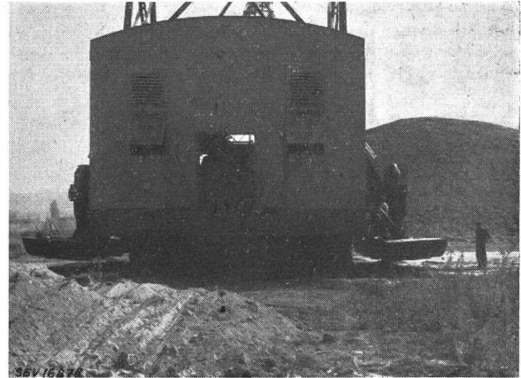
Fig. 5 Die Maschinenkabine des Baggers von hinten Links und rechts sieht man die beiden «Plattfüsse». Der Bagger ruht auf einer kreisförmigen, mit Roll-Lagern versehenen Platte
