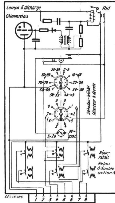
Fig. 2 Schema des Empfängers mit Dekadenwähler für 100 einfache Steuerbefehle Wahlkontakte 0...9: Einer-Reihe Wahlkontakte 0...99: Zehner-Reihe
