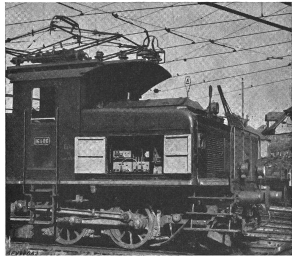
Fig. 2 Einbau der Rangierfunkapparate in eine Rangierlokomotive Unten rechts Umformer, daneben Sender und Empfänger, links oben Steuerzusatz mit auswechselbarem Nummernstöpsel
