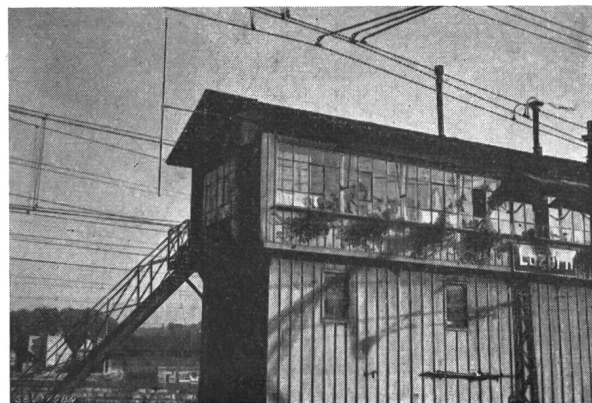
Fig. 3 Hauptstellwerk im Bahnhof Luzern Links oben die Antenne der drahtlosen Telephonanlage (Vertikaldipol)
