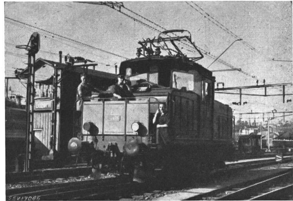
Fig. 6 Mit Rangierfunk ausgerüstete Rangierlokomotive Der Rangiermeister, Chef der Rangiergruppe, telephoniert während der Fahrt von der Lokomotive aus
