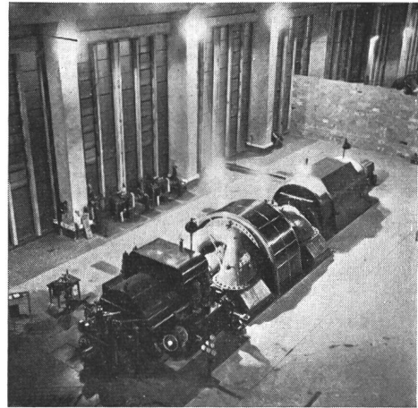
Fig. 3 50-MW-Turbogenerator (MFO/Escher-Wyss) des Kraftwerkes Dieppedalle
